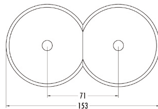
System pokrywający z dwiema ramkami.
