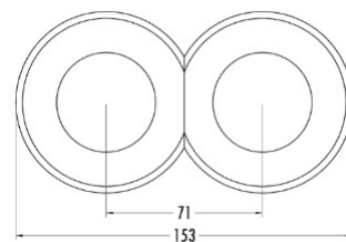
Ramki systemu z dwiema nakładkami dla centralnej wkładki.
