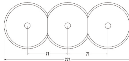
System pokrywający z trzema ramkami.
