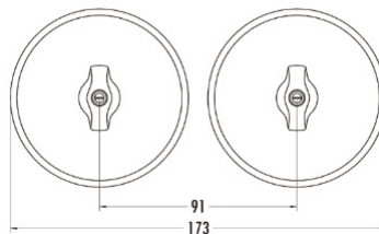
Ramki systemu z dwiema nakładkami dla centralnej wkładki.
